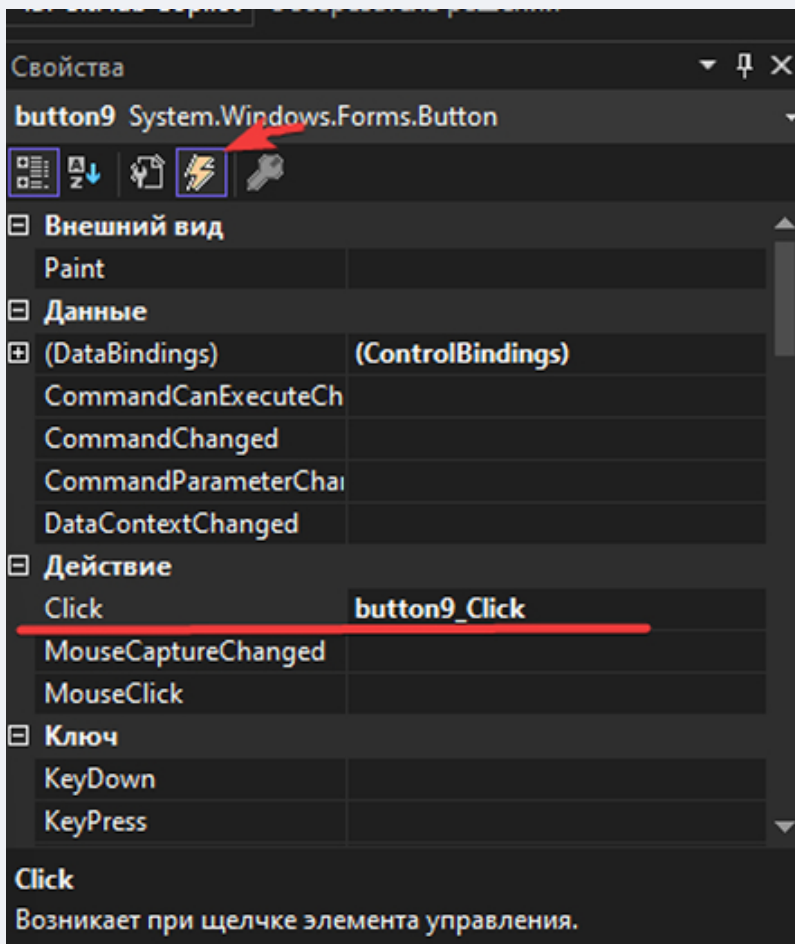
Рисунок 6.1 – Добавление событий
